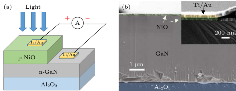
图 3 (a) 基于 NiO/GaN p-n 结的光电探测器结构示意图; (b) NiO/GaN p-n 结的截面 SEM 图, 插图为镀有电极的 p-n 结截面 SEM 放大图
